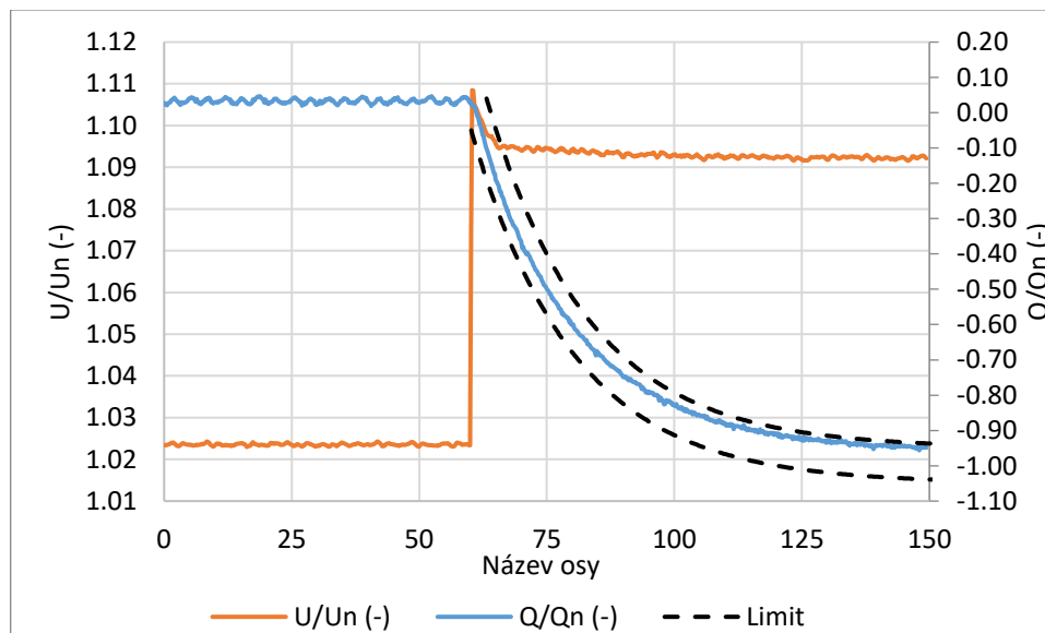
Obr.11.4: Q(U) – odezva Q na skokovou změnu U
