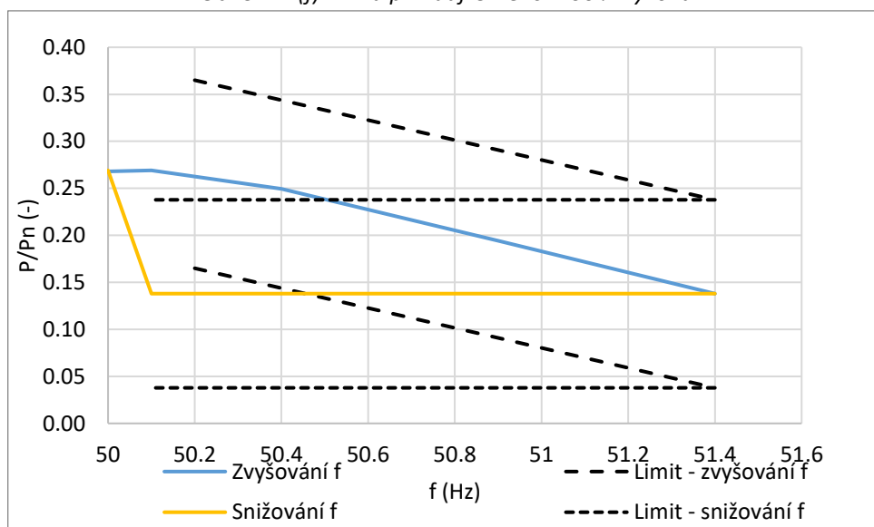
Obr.3.3: P(f) křivka při nadfrekvenci – 25 % výkonu
