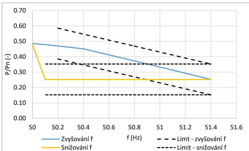
Obr.3.2: P(f) křivka při nadfrekvenci – 50 % výkonu
