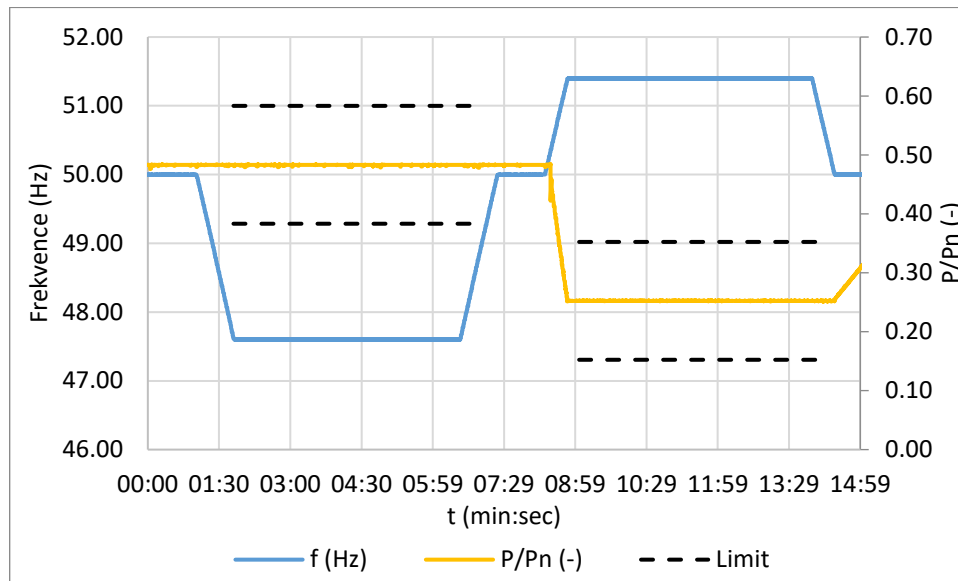
Obr.1.1: Frekvenční stabilita
